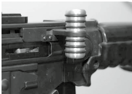
Figura 18: Leva d'armamento anatomica per F ass 57
