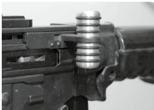
Bild 18: Ladegriff anatomisch zu Stgw 57
